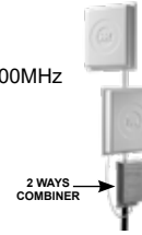
5 COL2 4-bands 800 - 900 - 1800 - 2100MHz
