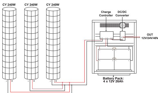
Cabinet CAB Dim. 540 x 230 x 650mm
